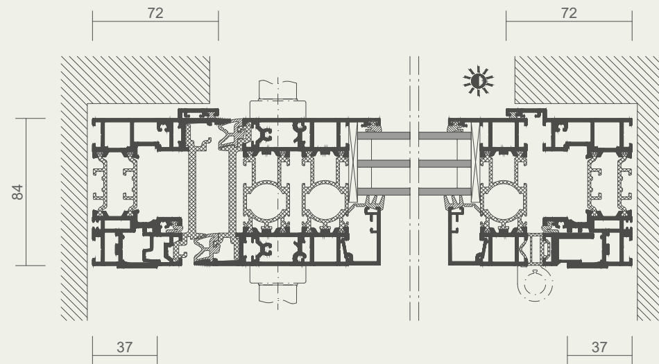
Horizontalschnitt
