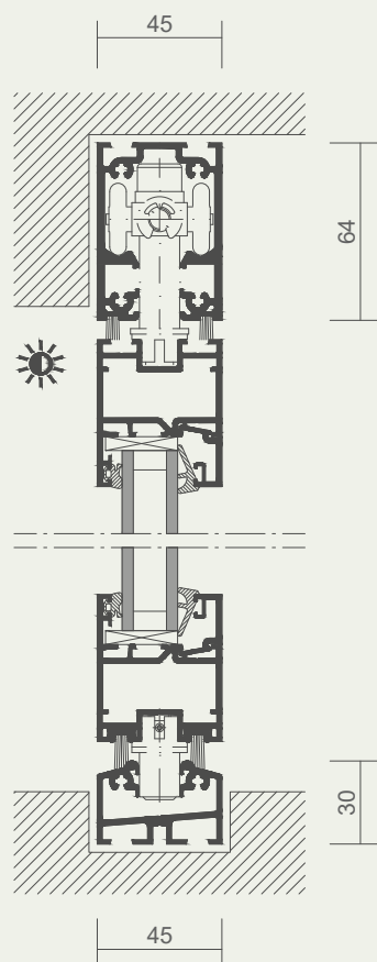
Vertikalschnitt
