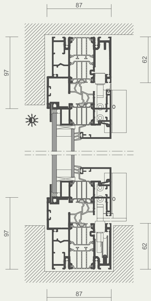
Vertikalschnitt
