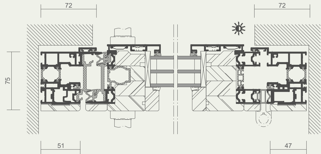
Horizontalschnitt
