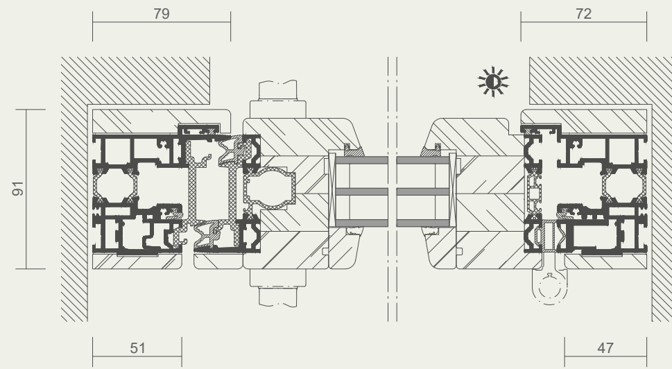
Horizontalschnitt
