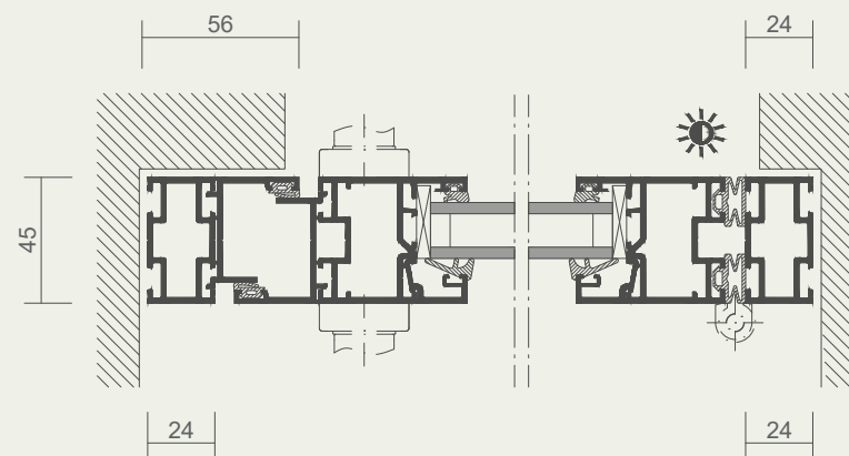
Horizontalschnitt
