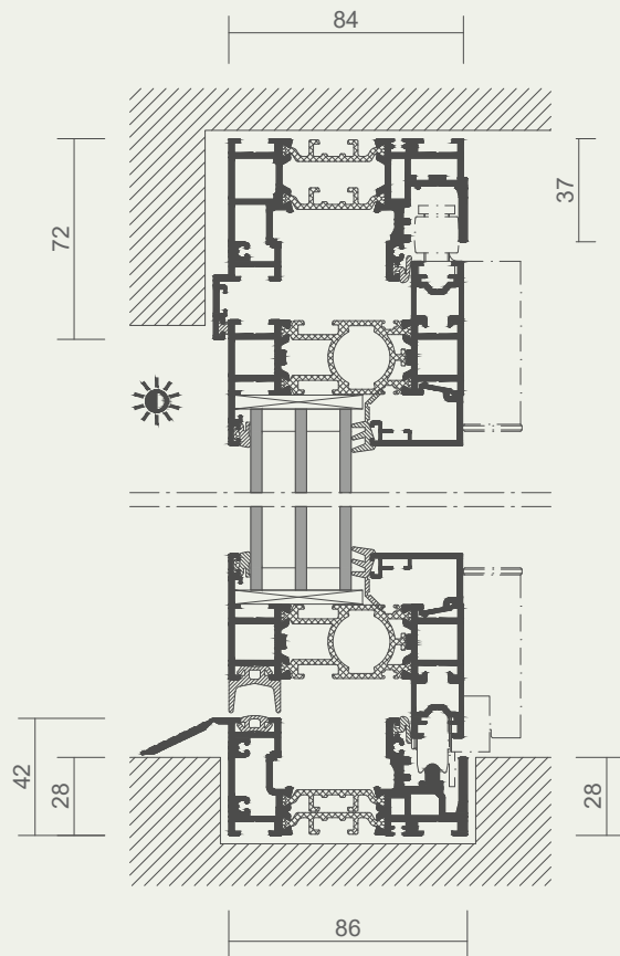
Vertikalschnitt
