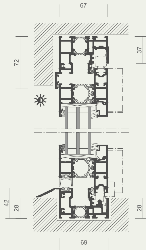
Vertikalschnitt
