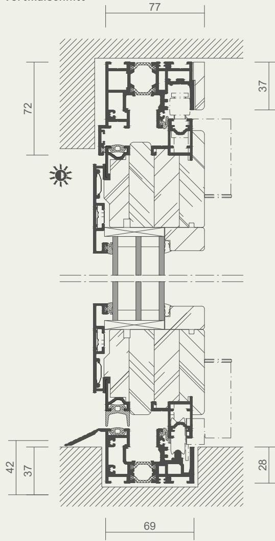
Vertikalschnitt
